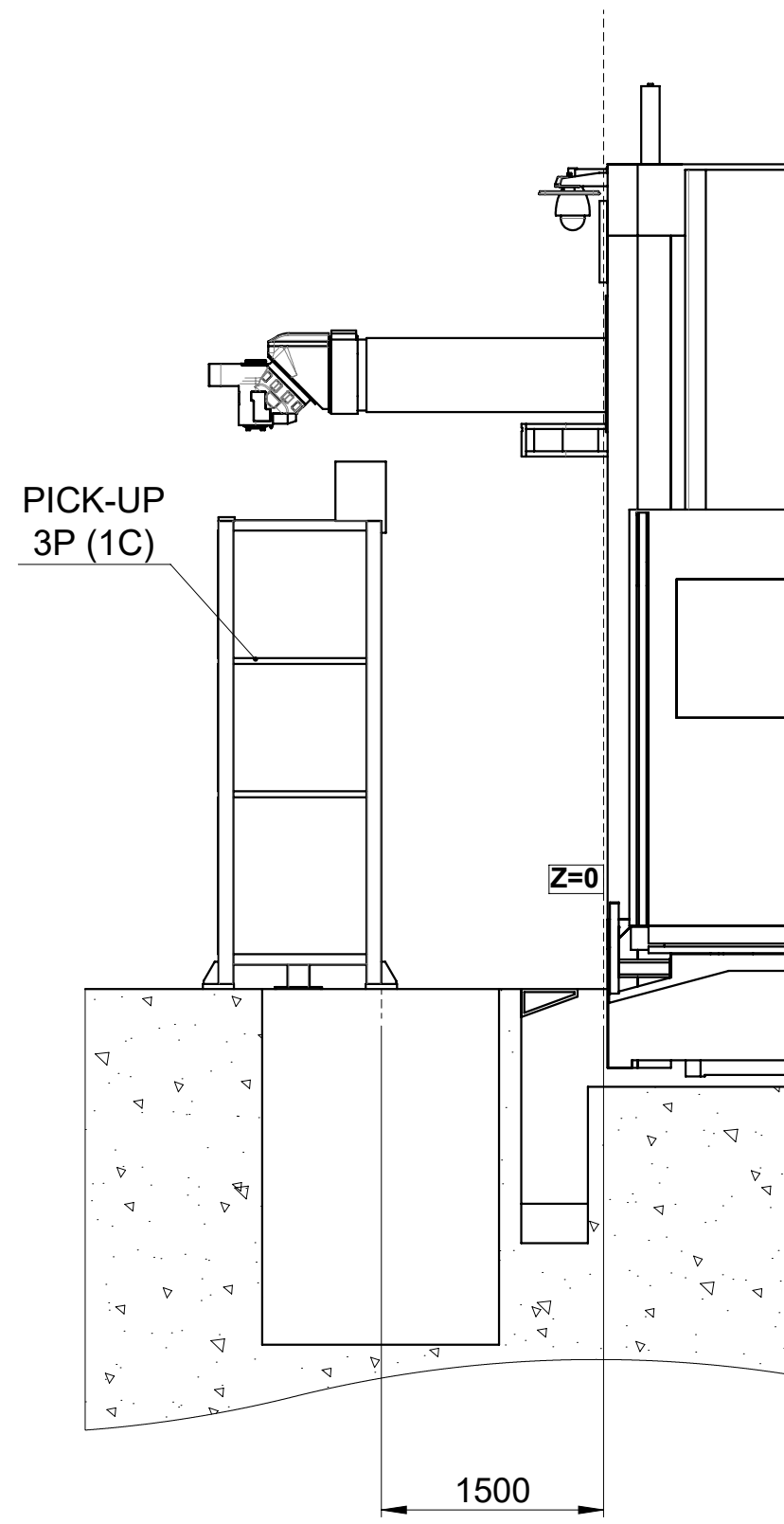
A-A 270°
